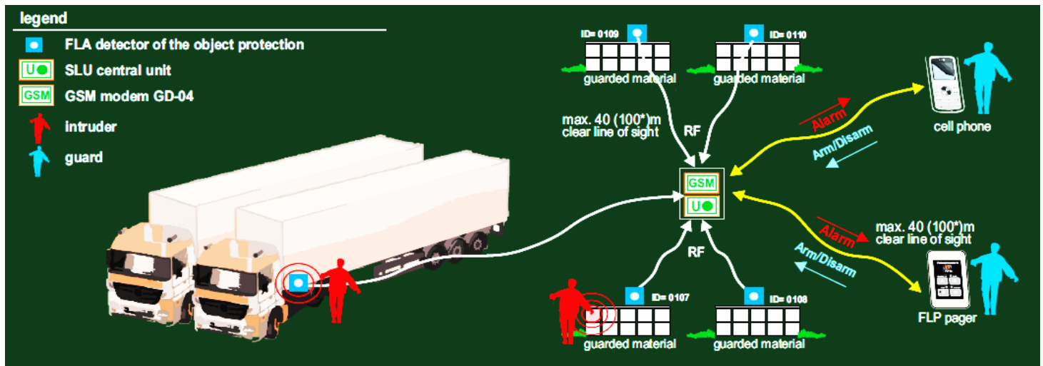
Systemarchitektur mit GSM- Modem – Radius bis zu 50m
