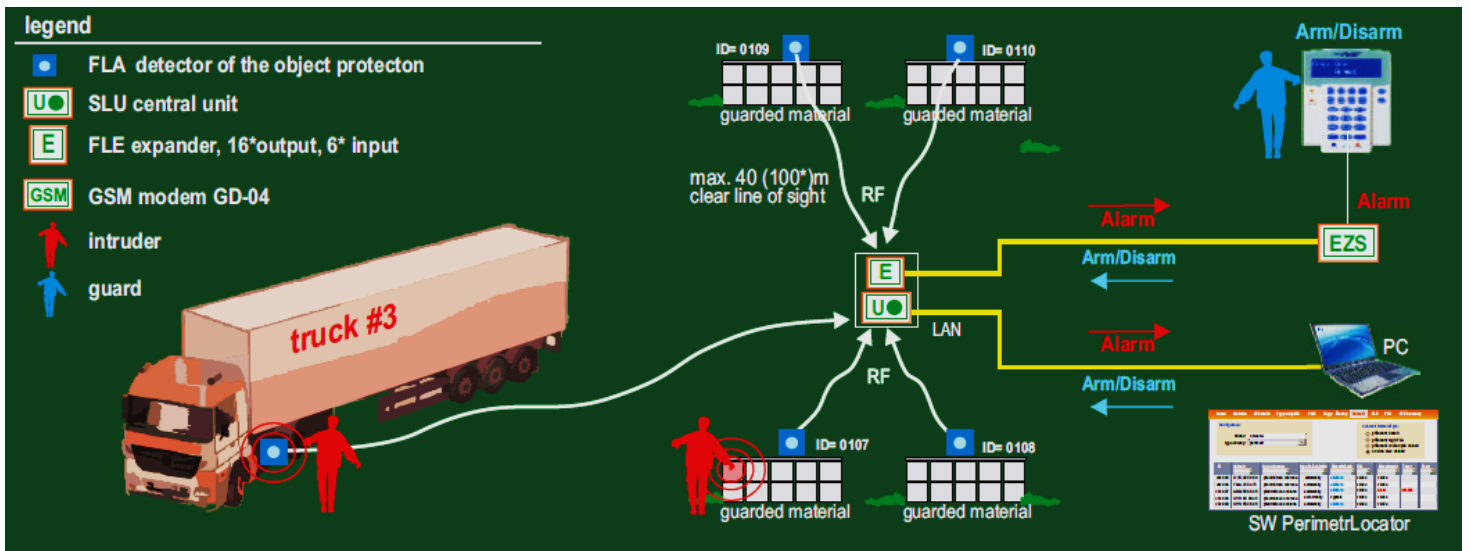
Systemarchitektur mit einer Einbruchmeldeanlage
