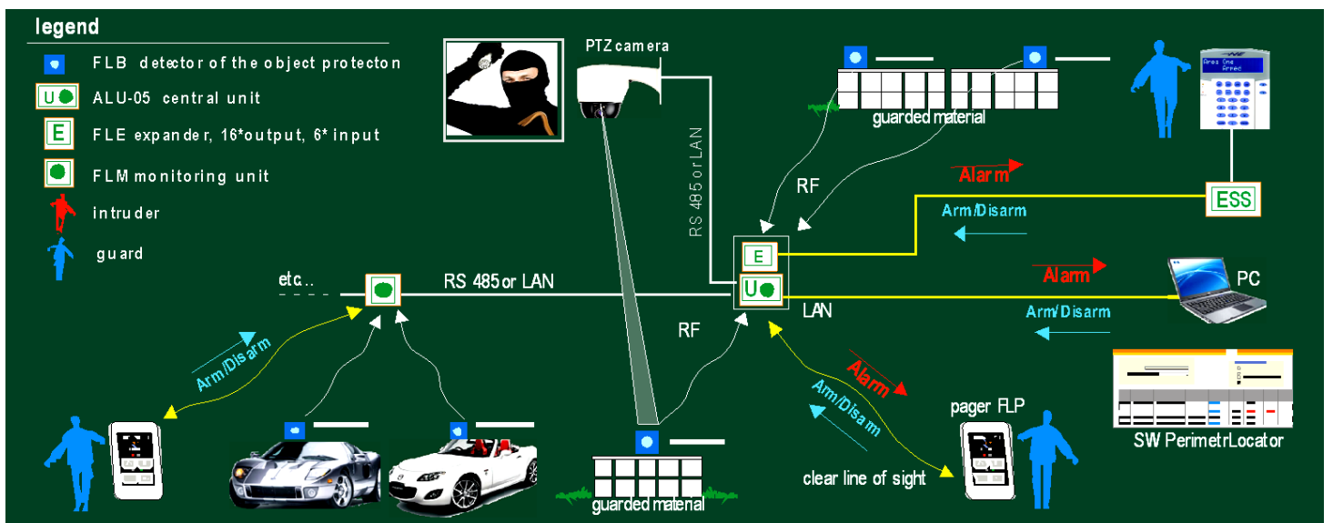
Systemarchitektur mit Computer oder Alarmanlage und mehreren FLM Einheiten
